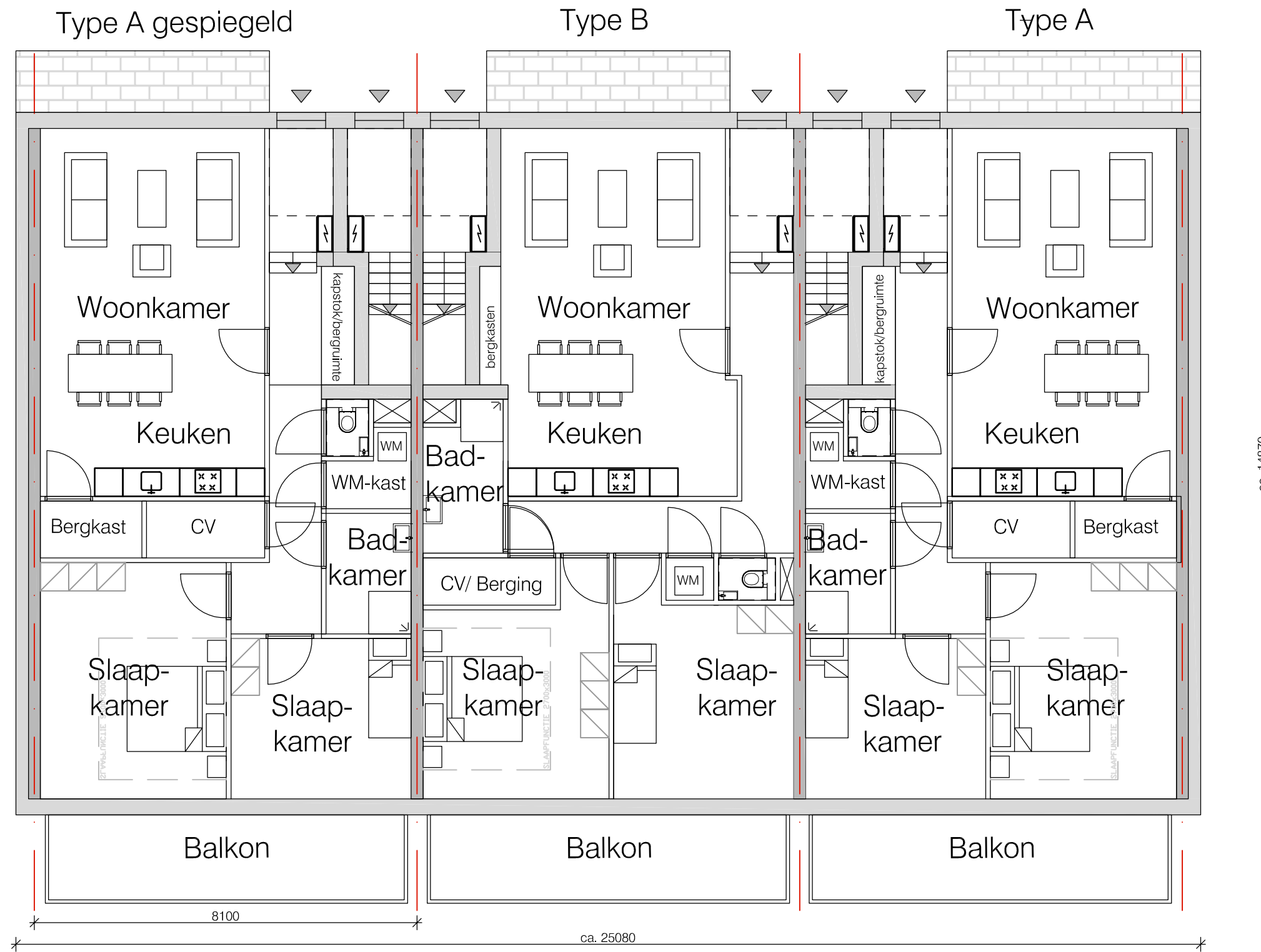
Plattegrond begane grond
