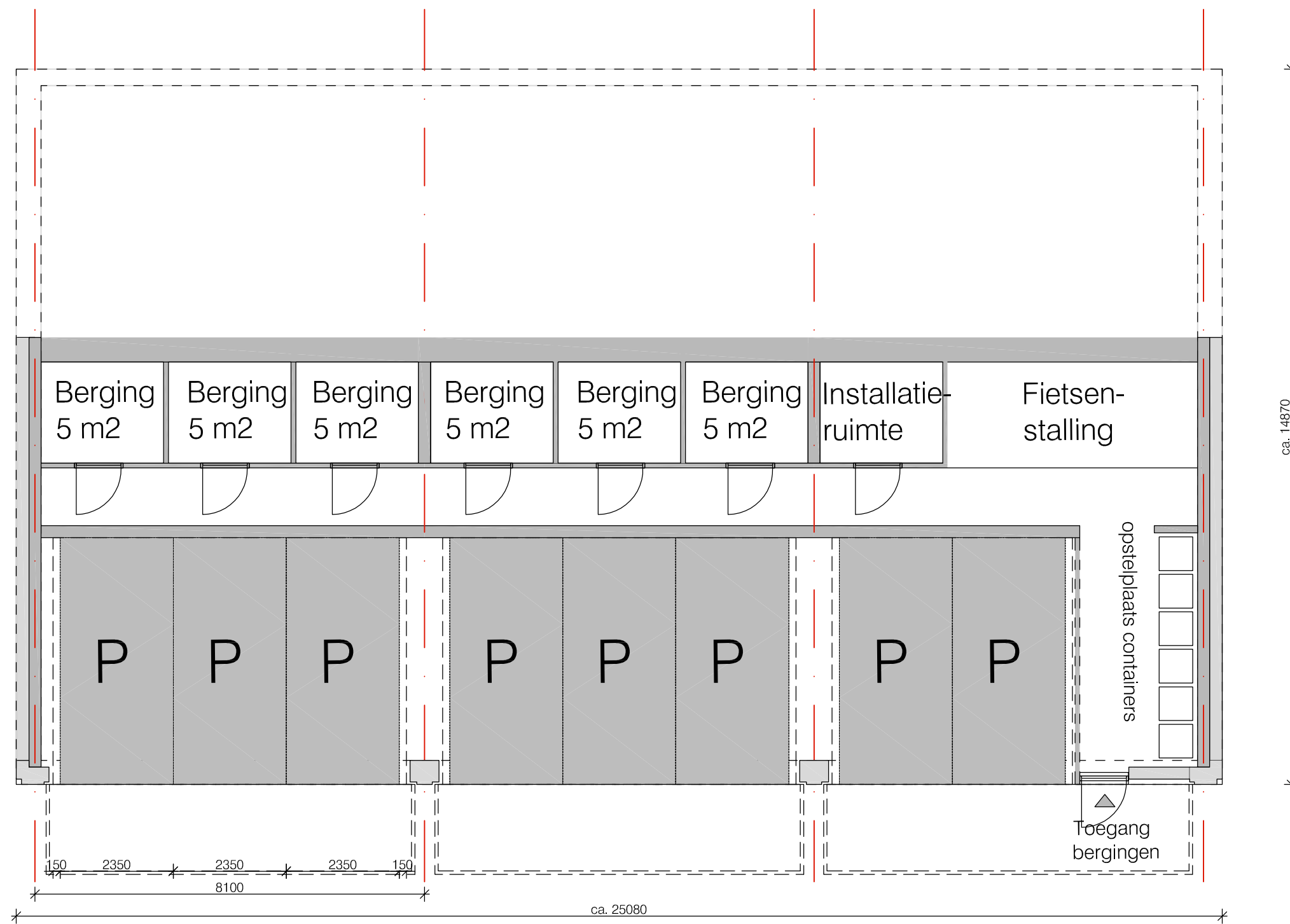
Plattegrond souterrain / terrein
