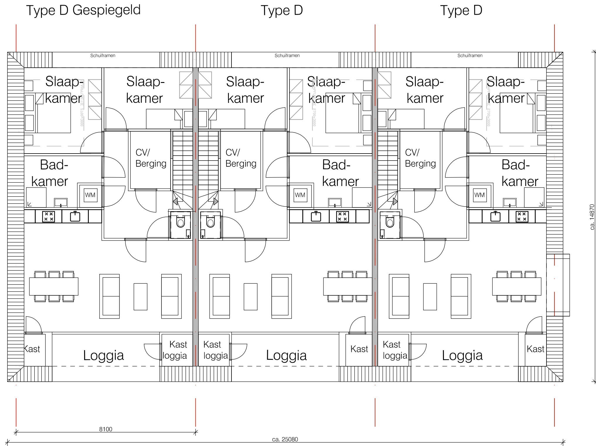
Plattegrond 1e verdieping
