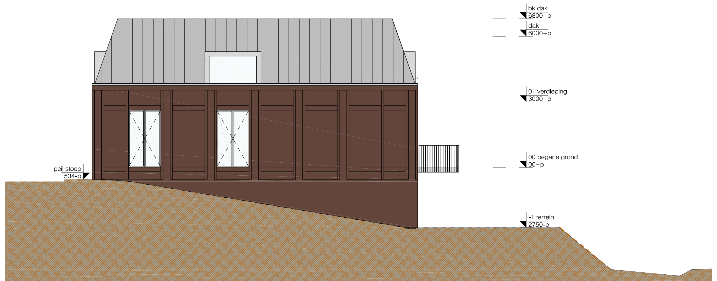
Gevel rechts
