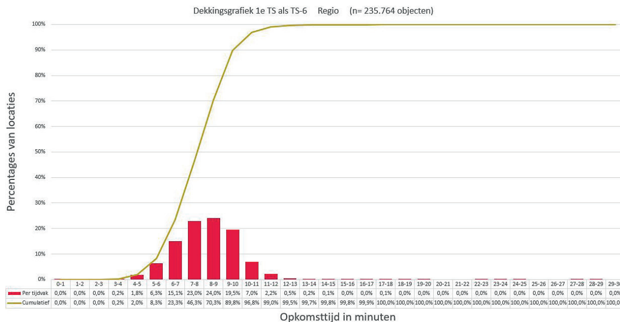
Dekkingsgrafiek snelheid basiseenheid TS met 6 personen
