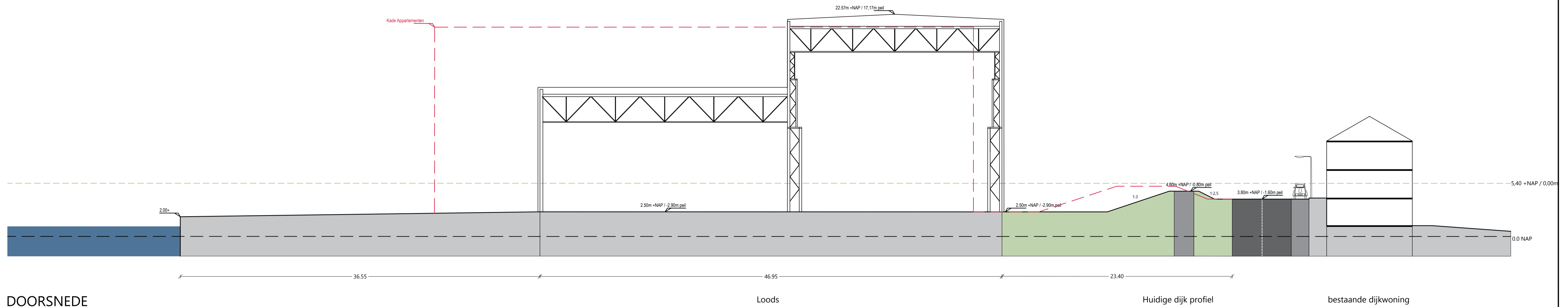
DOORSNEDE Bestaande situatie
