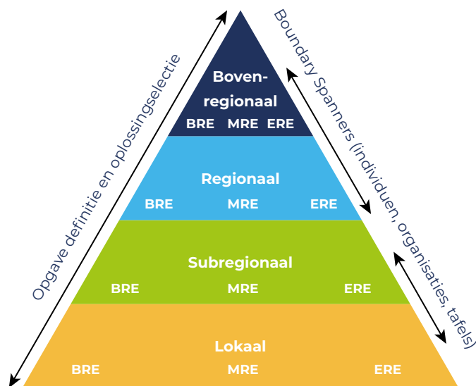
Figuur 5 Weergave van een ‘volwassen’ samenspel tussen BRE, MRE en ERE, waarin de verschillende schaalniveaus elkaar versterken.
